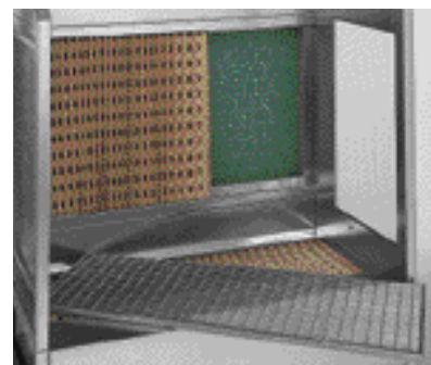
En cas de besoin, les moyens filtrants, le préfiltre et le filtre fin se remplacent en un tournemain.
